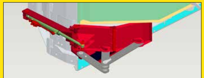
Strooikap met strooibegrenzingsluik(en)
